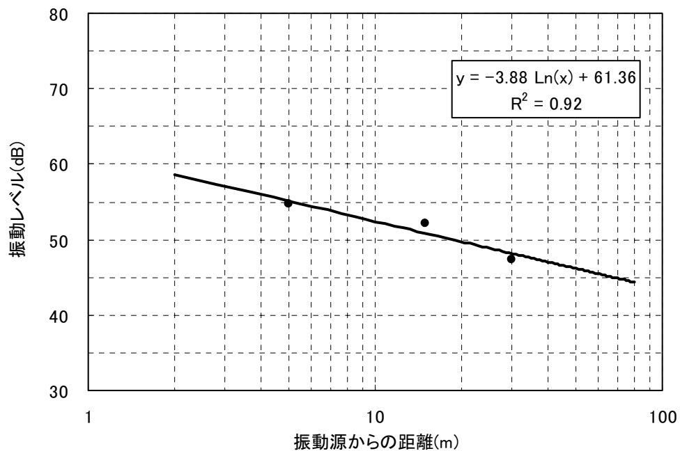
図2 振動の距離減衰
