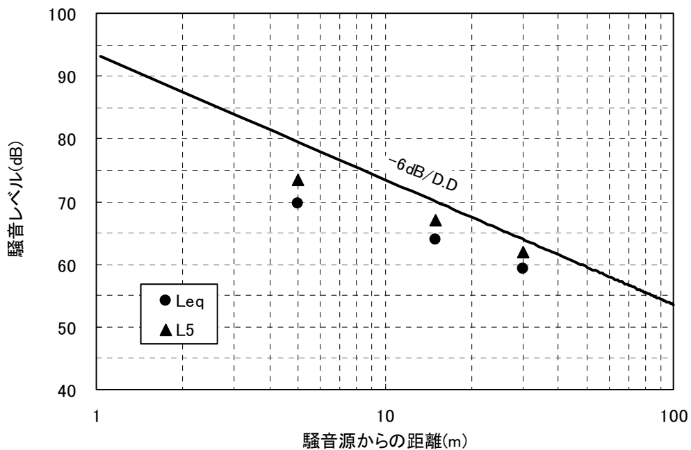
図1 騒音の距離減衰
